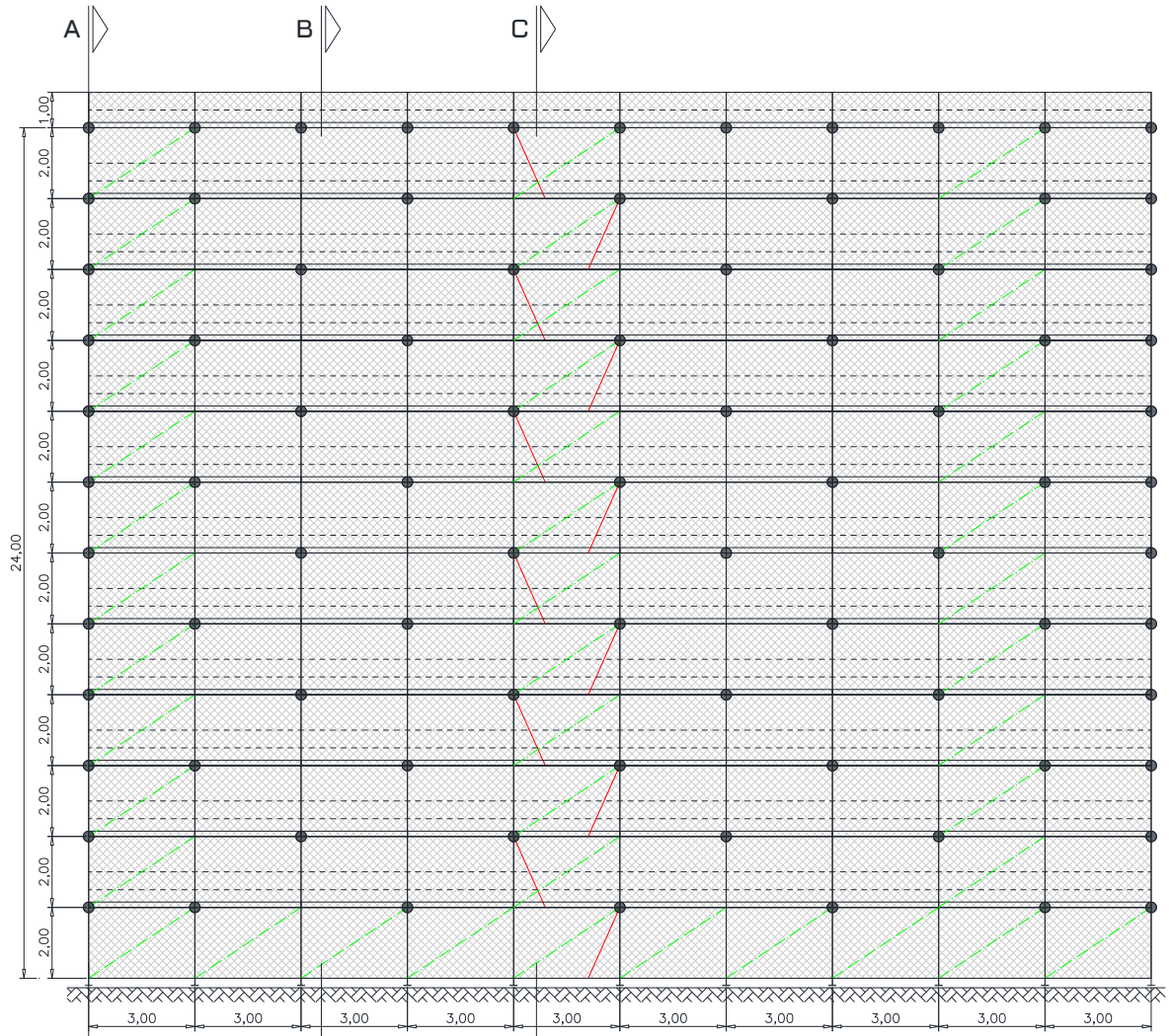
Elevation
